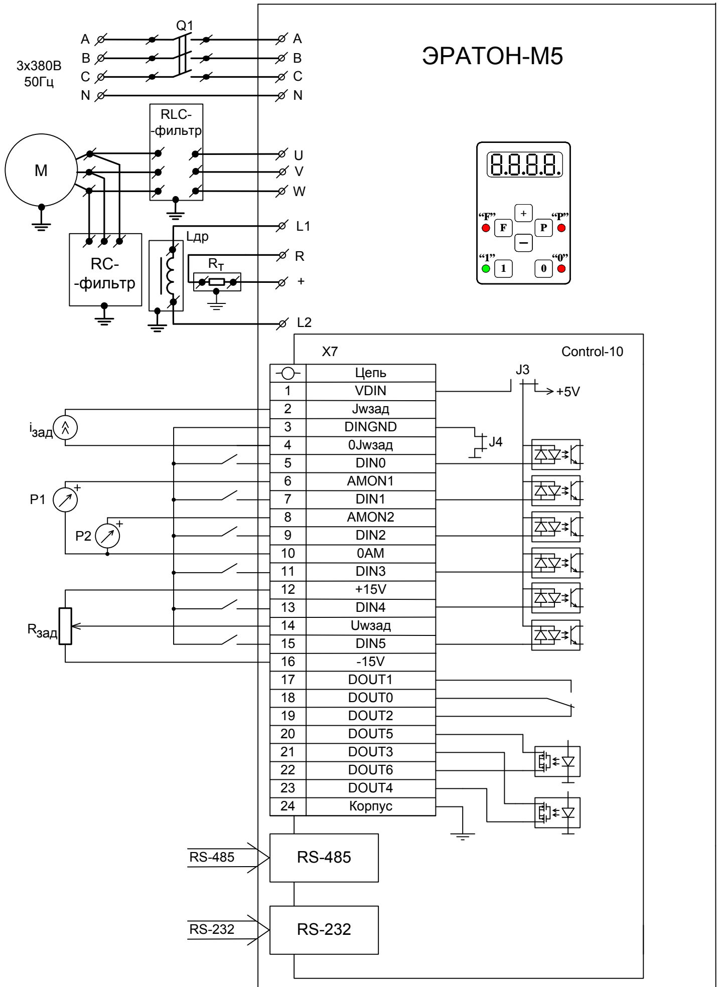
Схема электрическая общая электропривода
