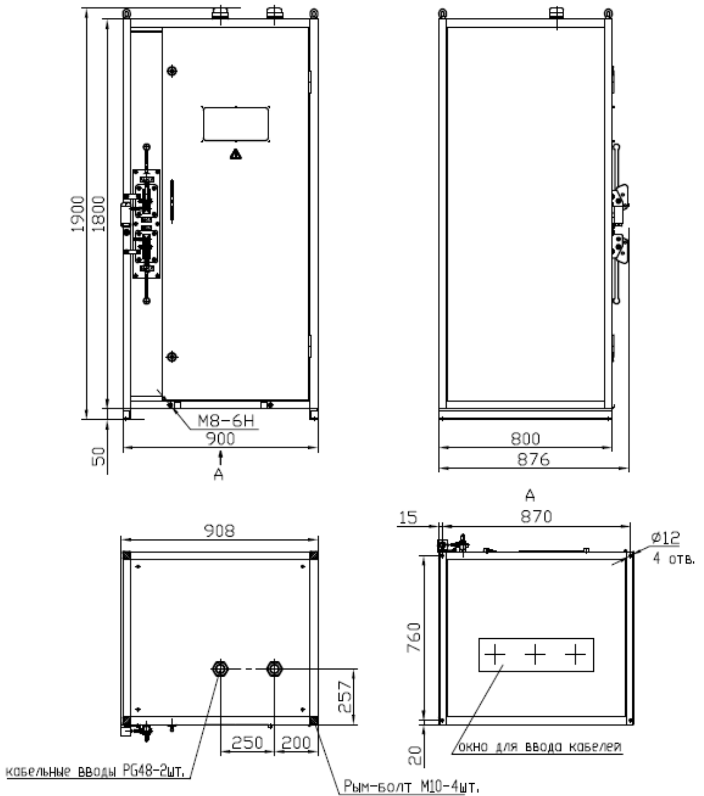
Рисунок Б.1 – Габаритные и установочные размеры КРУ-6-01
