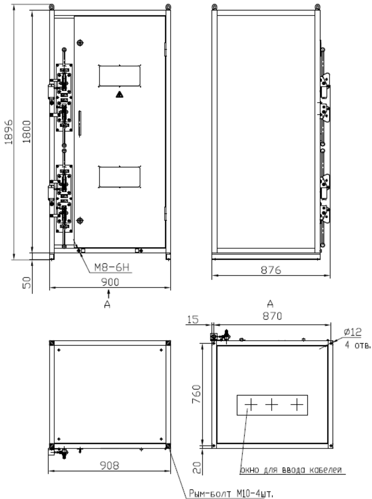
Рисунок Б.4 – Габаритные и установочные размеры КРУ-6-03
