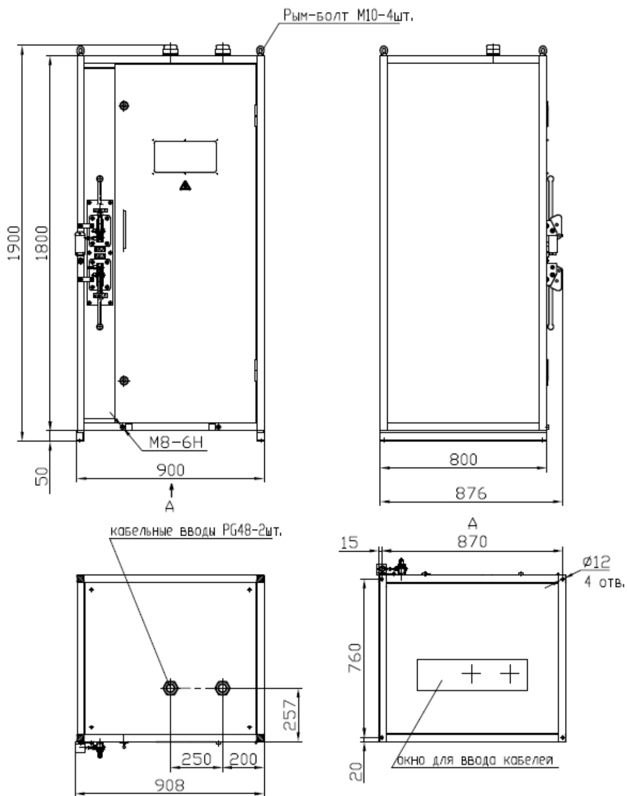
Рисунок Б.2 – Габаритные и установочные размеры КРУ-6-02-80, КРУ-6-02-100, КРУ-6-02-160
