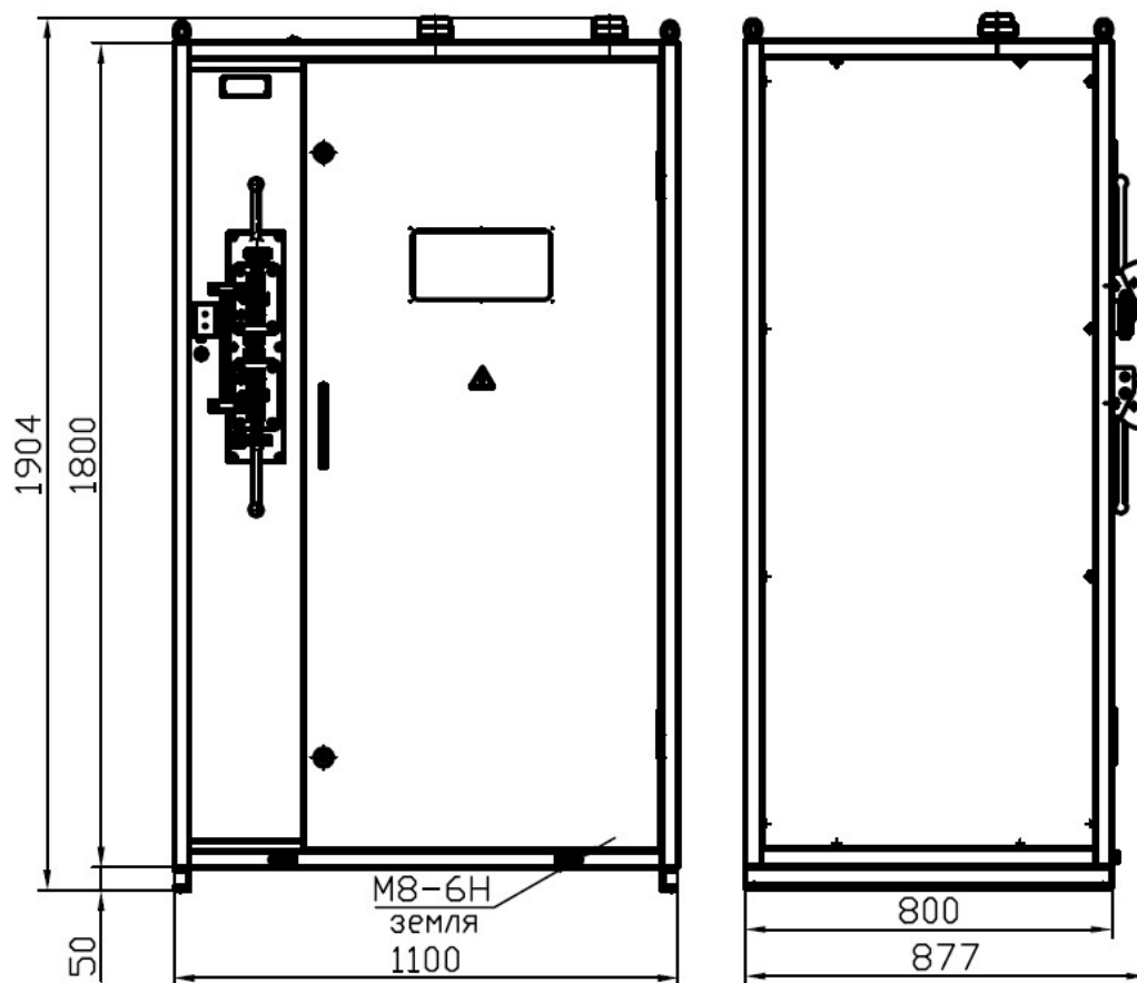
Рисунок В.4 – Габаритные размеры КРУ-6-04
