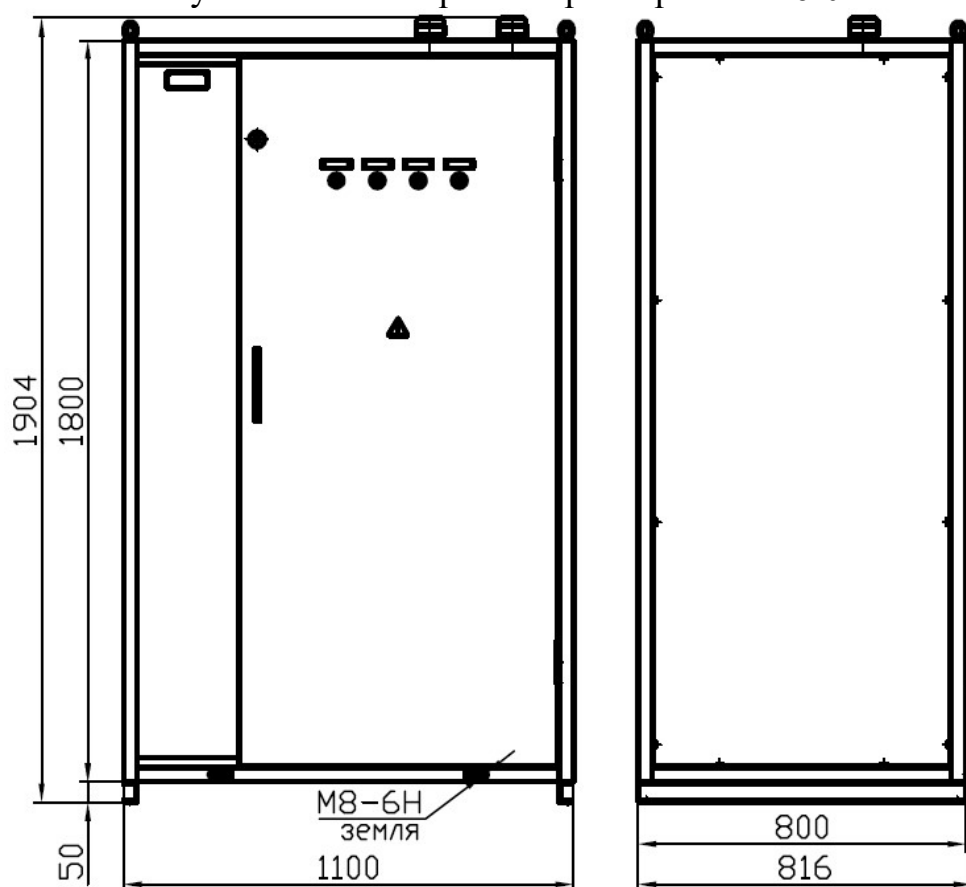
Рисунок В.4 – Габаритные размеры КРУ-6-04
