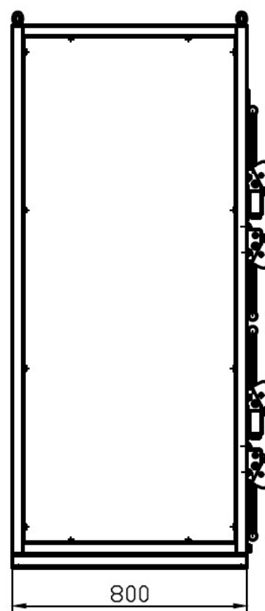
Рисунок В.2 – Габаритные размеры КРУ-6-02
