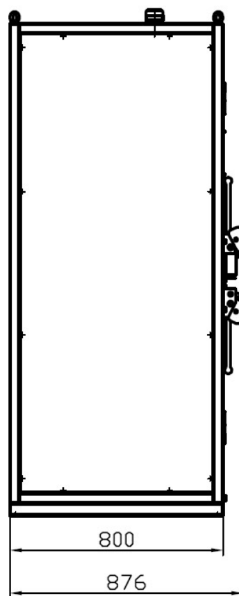
Рисунок В.2 – Габаритные размеры КРУ-6-02
