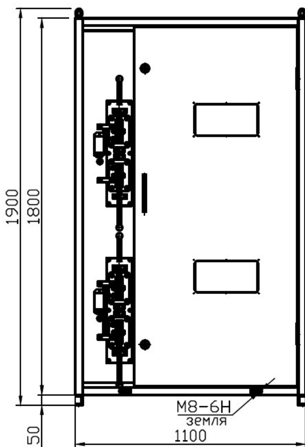
Рисунок В.2 – Габаритные размеры КРУ-6-02
