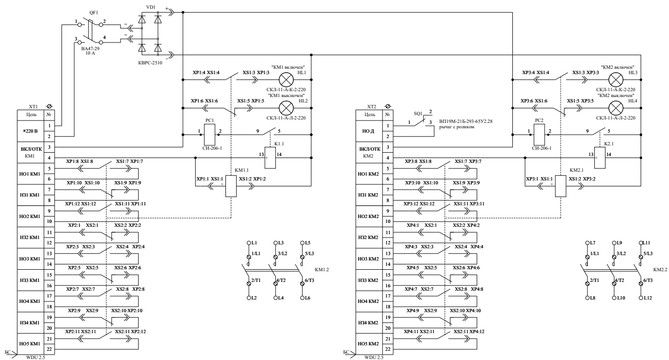
Рисунок Б.5 – Схема электрическая принципиальная КРУ-6-05
