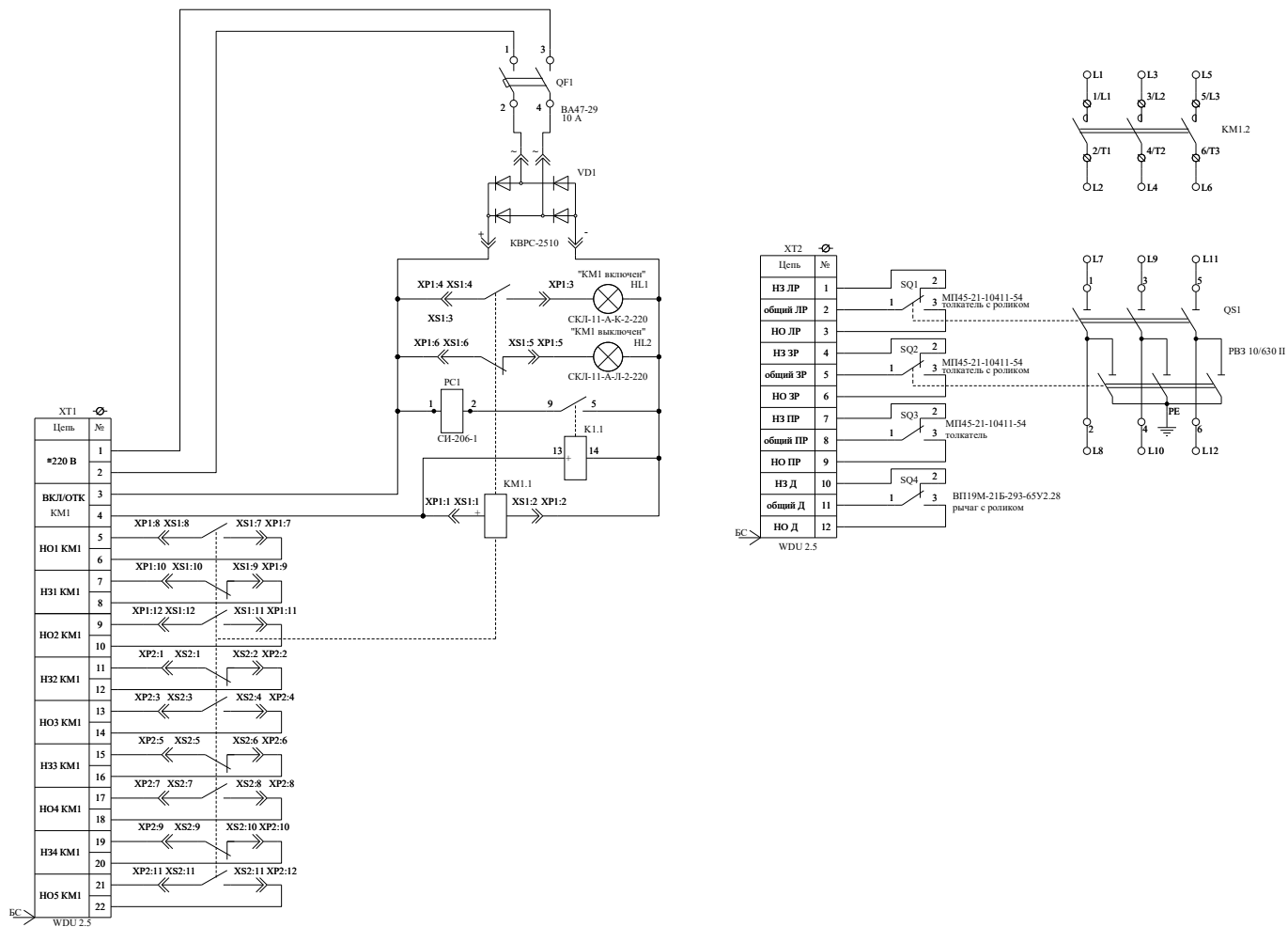
Рисунок Б.4 – Схема электрическая принципиальная КРУ-6-04
