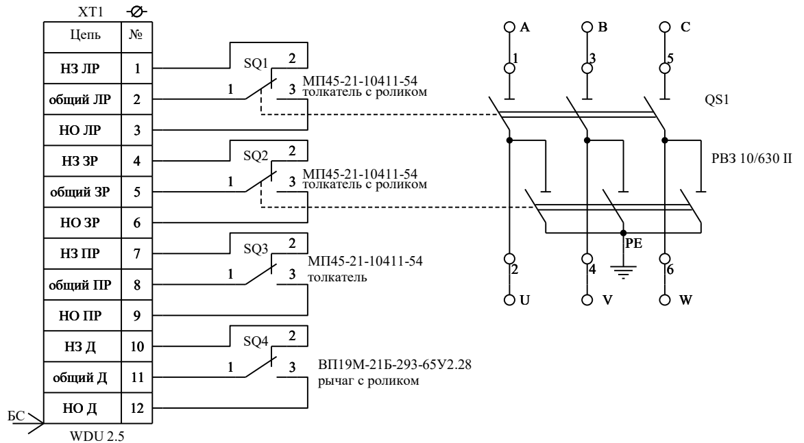
Рисунок Б.1 – Схема электрическая принципиальная КРУ-6-01
