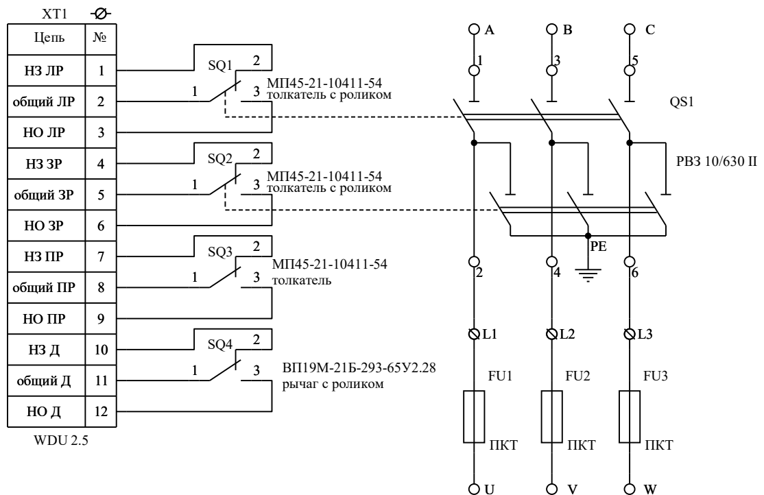
Рисунок Б.2 – Схема электрическая принципиальная КРУ-6-02
