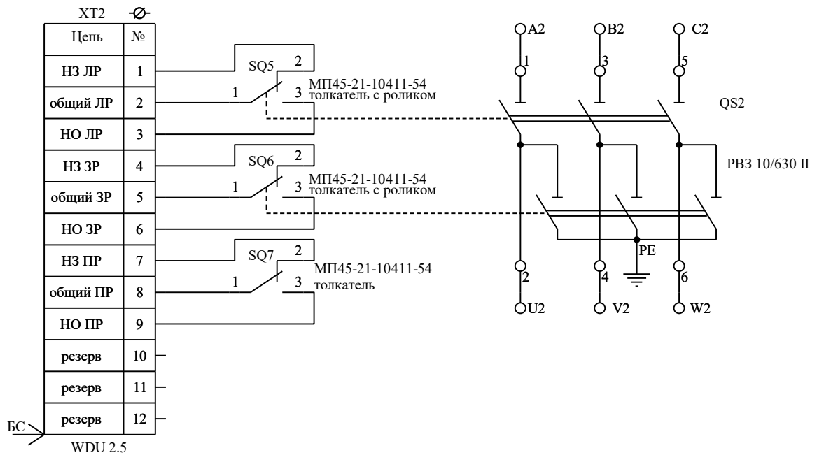
Рисунок Б.3 – Схема электрическая принципиальная КРУ-6-03
