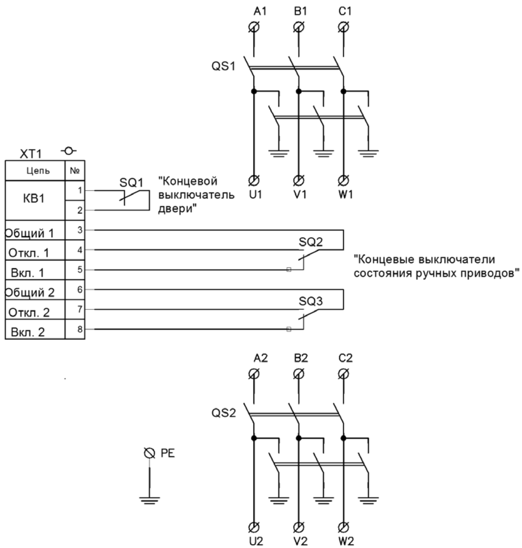
Рисунок А.3 – Схема электрическая принципиальная КРУ-6-03
