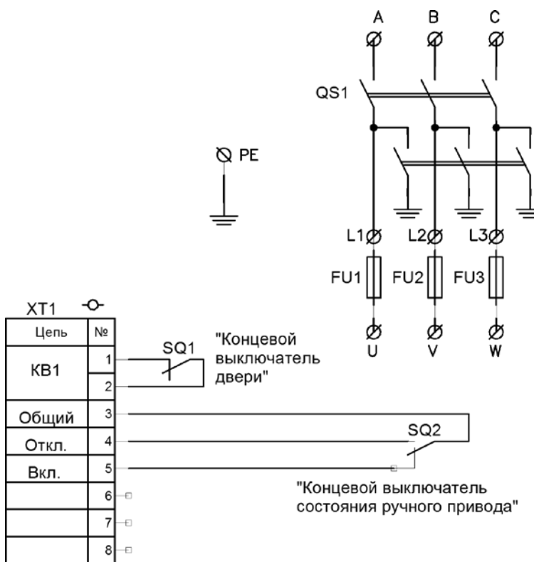
Рисунок А.1 – Схема электрическая принципиальная КРУ-6-01
