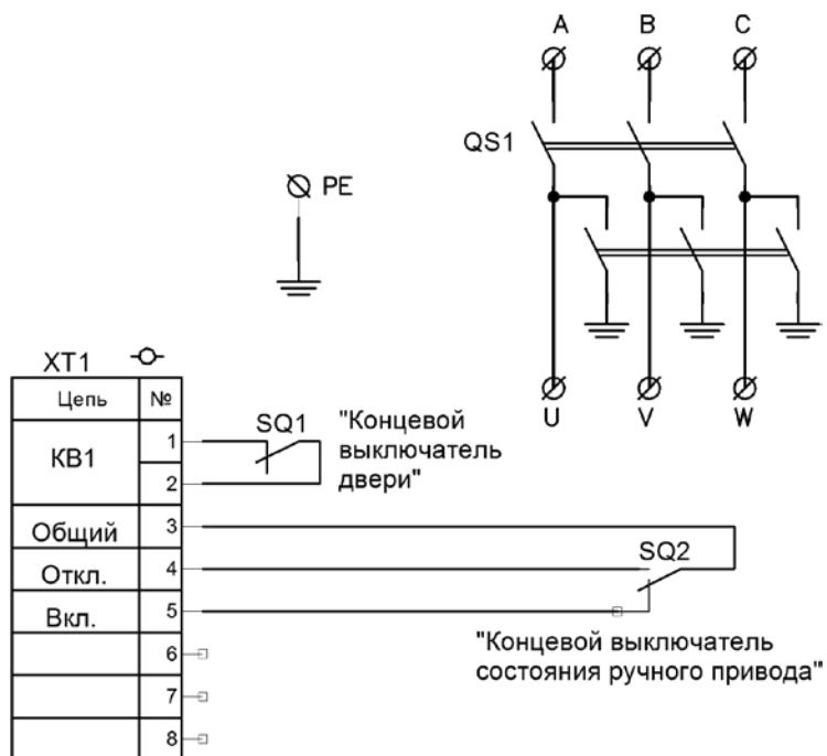
Рисунок А.1 – Схема электрическая принципиальная КРУ-6-01
